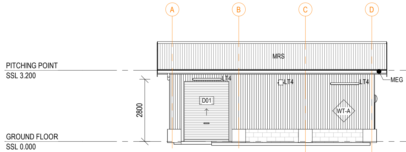
A 300 ELEVATION SCALE : 1 : 100
