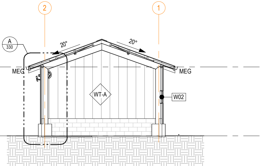
F 300 SECTION SCALE : 1 : 100
