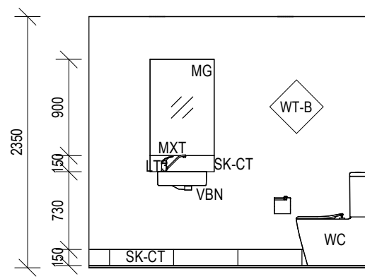
E 311 ELEVATION SCALE : 1 : 50
