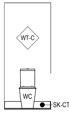
F 311 ELEVATION SCALE : 1 : 50
