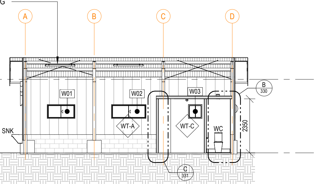
E 300 SECTION SCALE : 1 : 100
