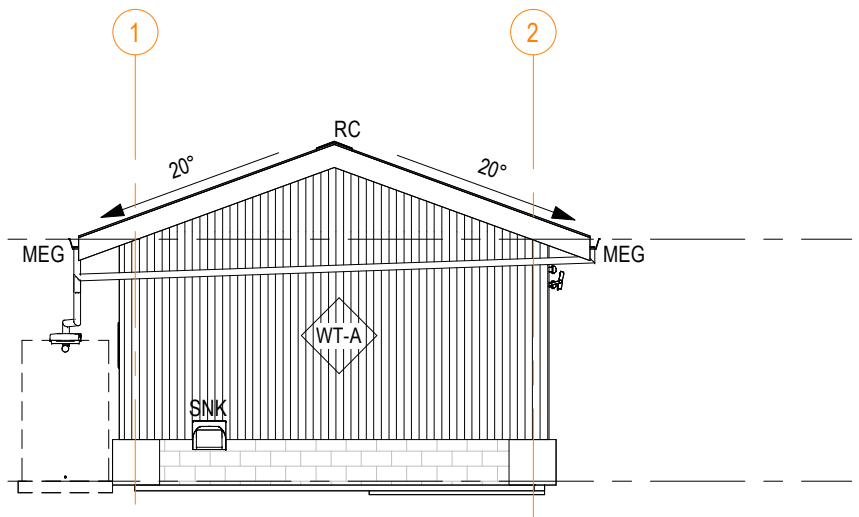
B 300 ELEVATION SCALE : 1 : 100
