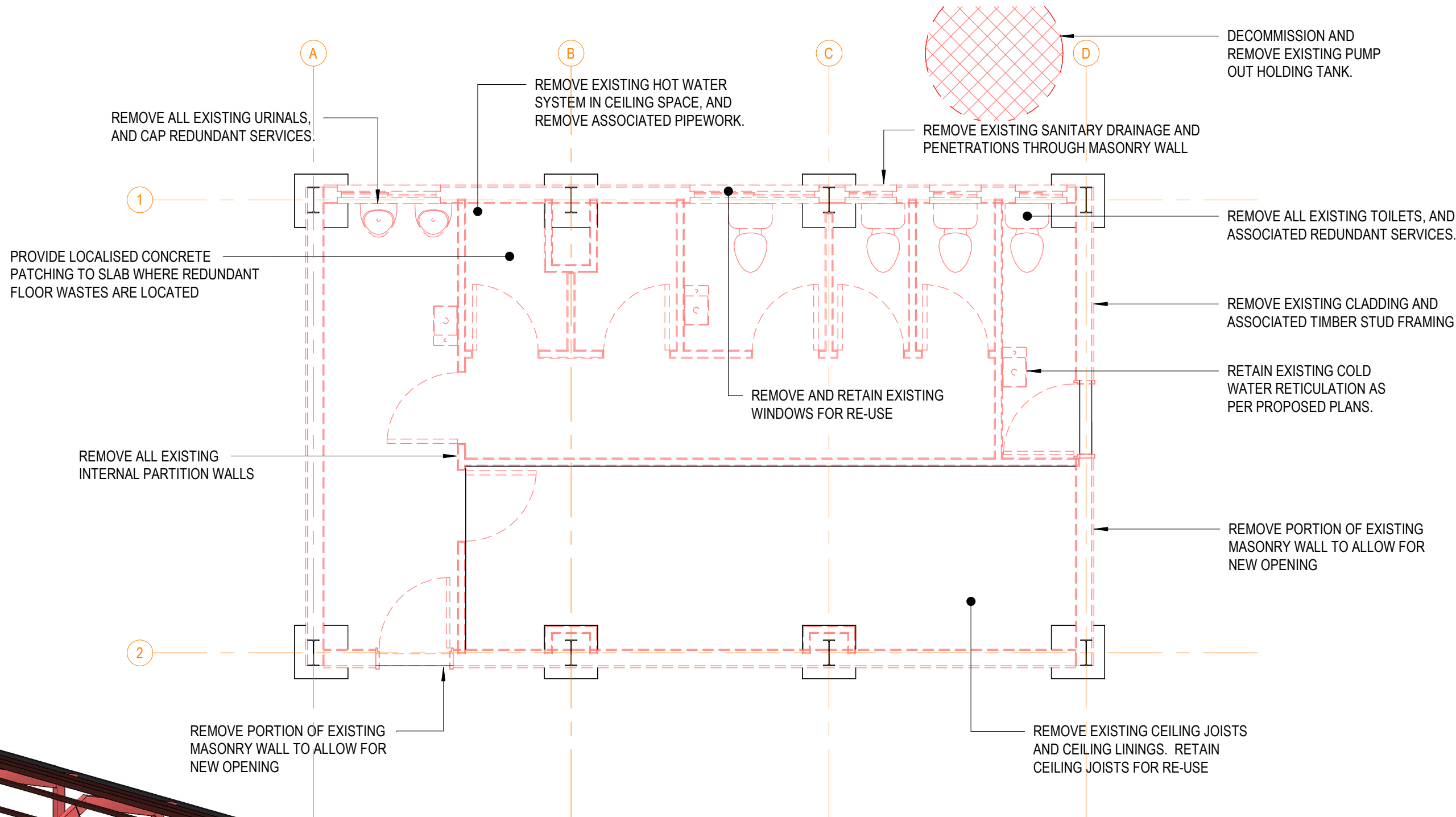
DEMOLITION PLAN SCALE : 1 : 50
