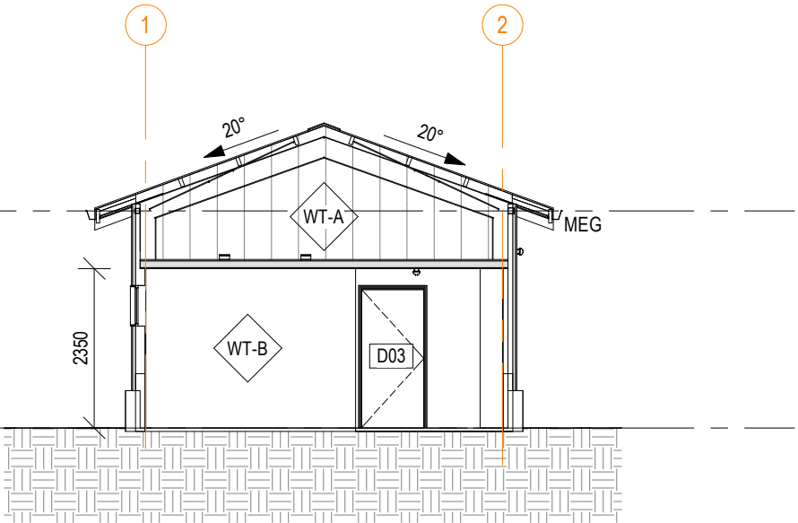
G 300 SECTION SCALE : 1 : 100
