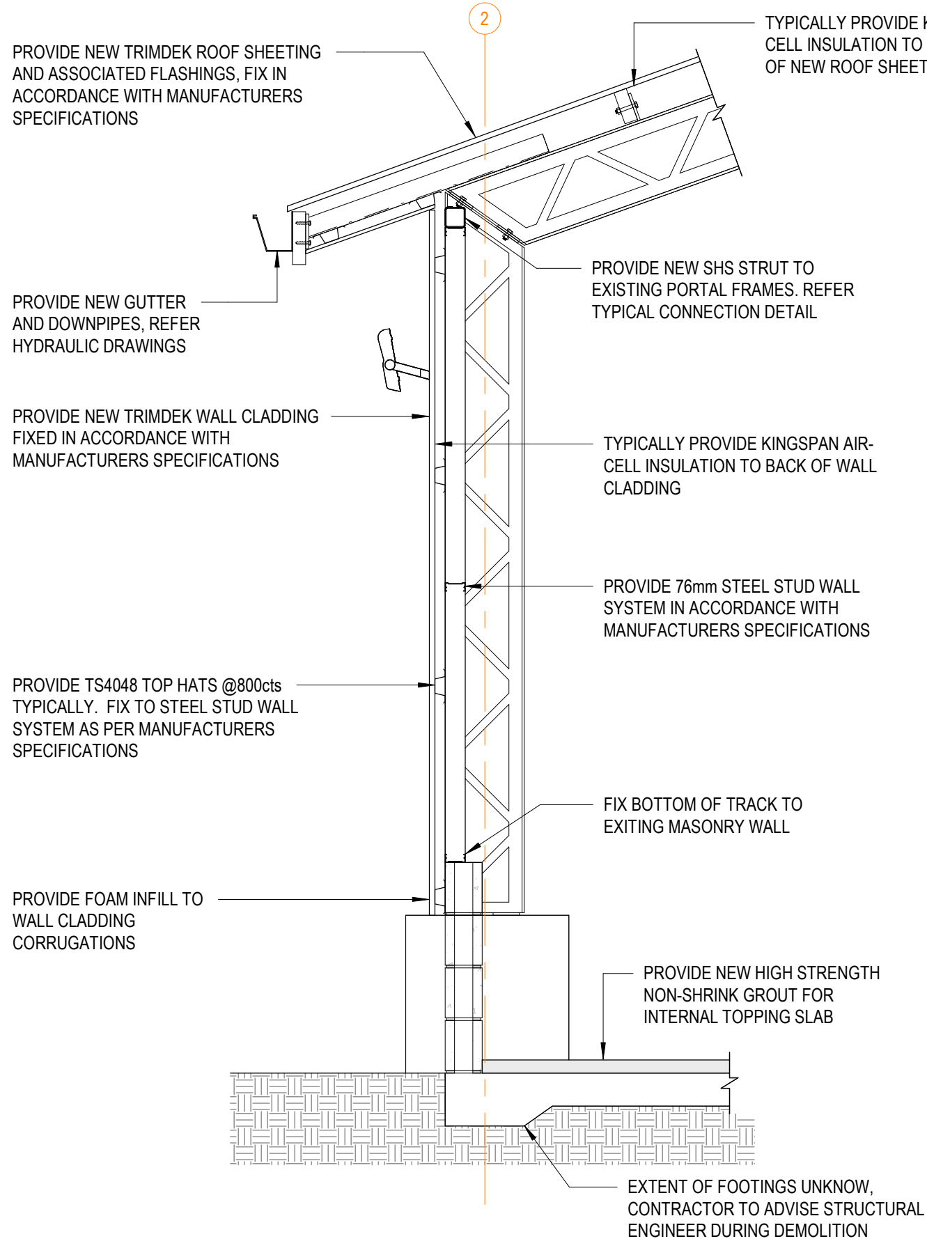
A 312 DETAIL SCALE : 1 : 20
