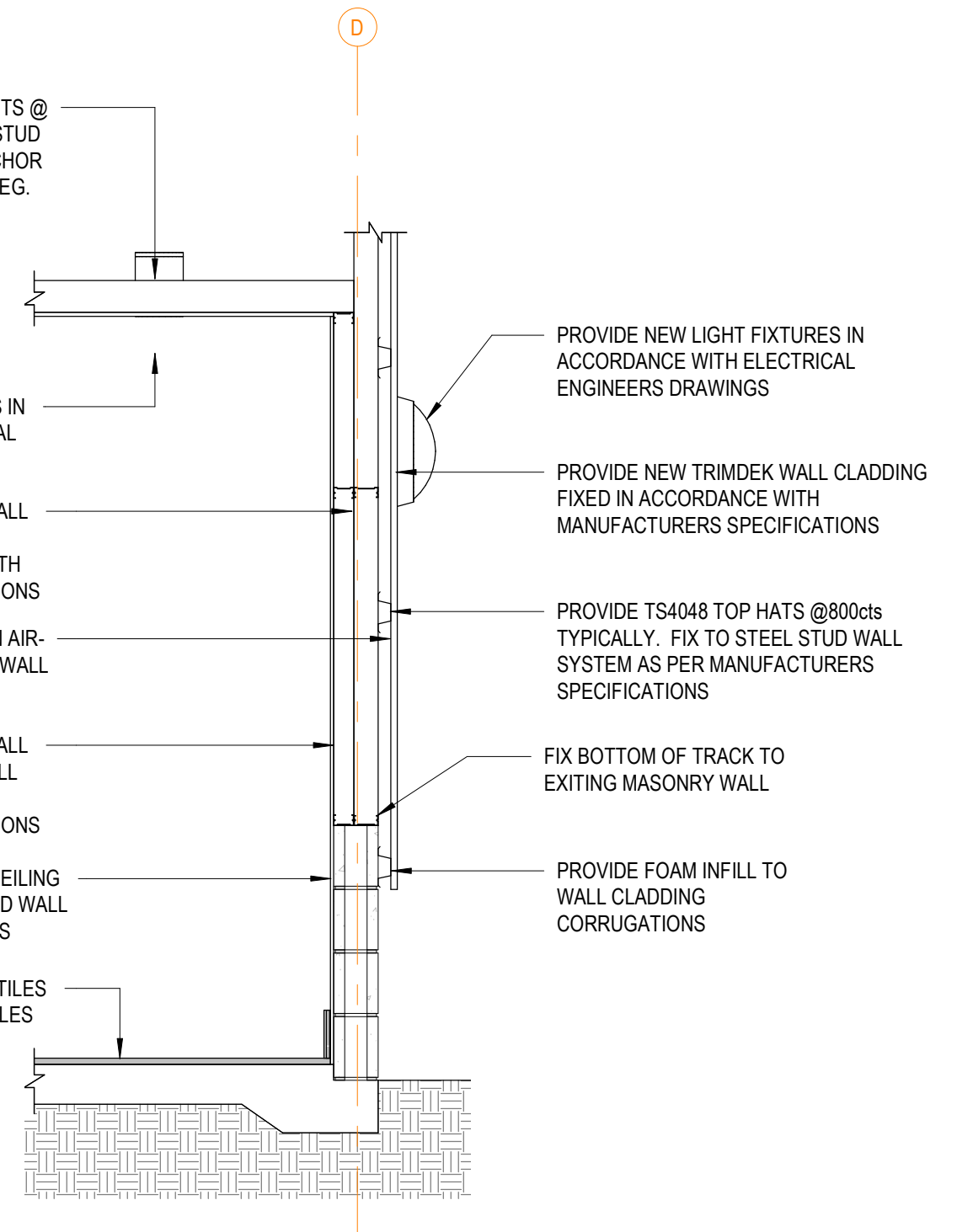
B 312 DETAIL SCALE : 1 : 20
