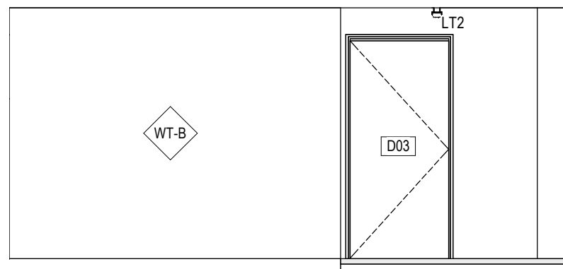
C 311 ELEVATION SCALE : 1 : 50
