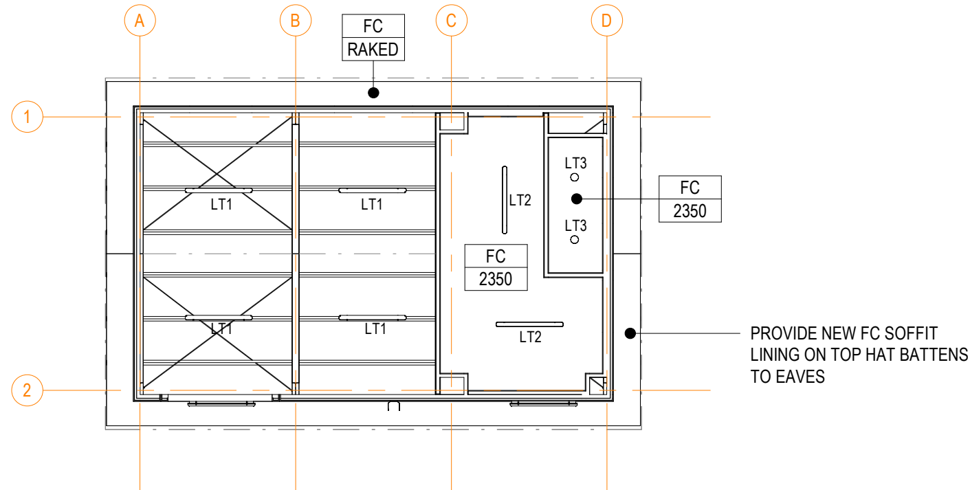
REFLECTIVE CEILING PLAN SCALE : 1 : 100
